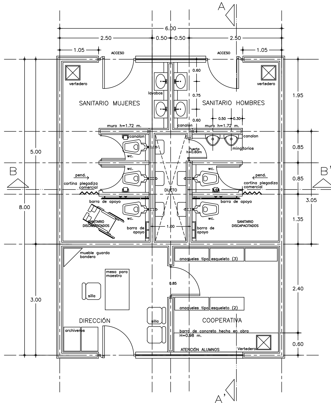
PLANTA ARQUITECTONICA
