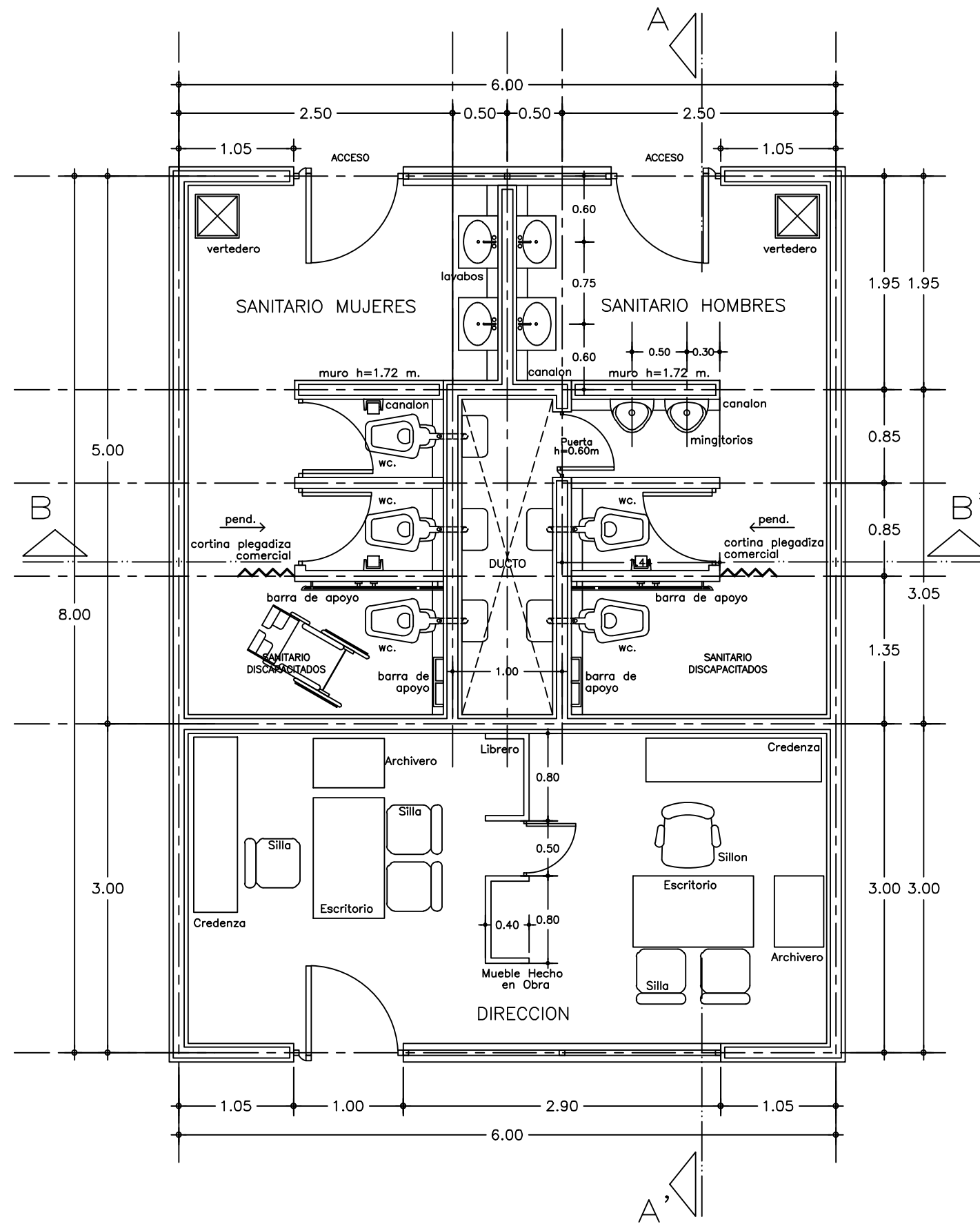
PLANTA ARQUITECTONICA
