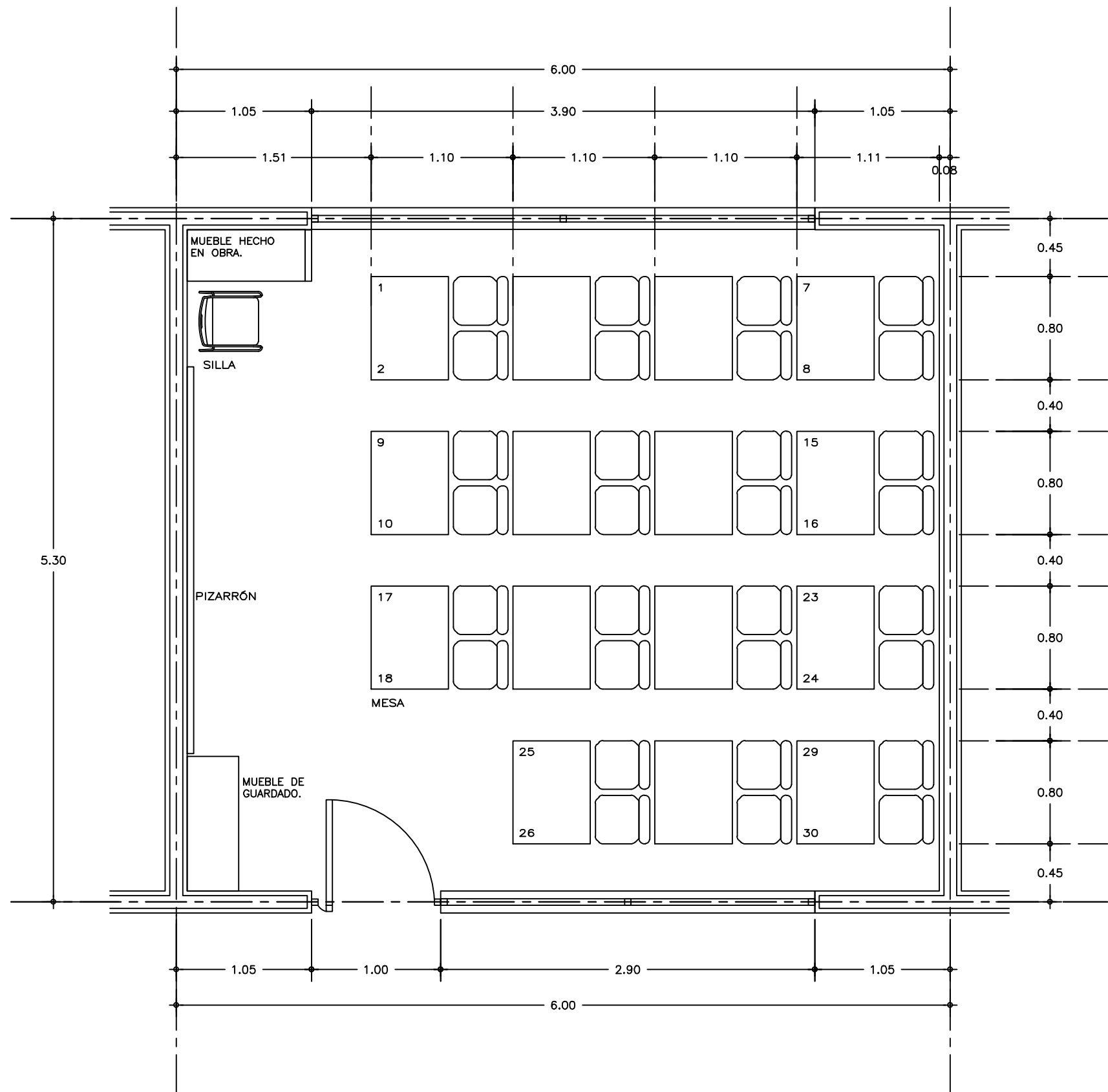
PLANTA ARQUITECTONICA AULA DE 6.00x5.30 M. CAP. 30 ALUMNOS (JARDIN DE NIÑOS)
